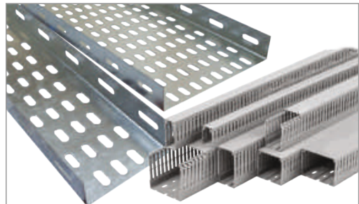
Cable Ducts & Trays Kablo Kanalları ve Tavaları
